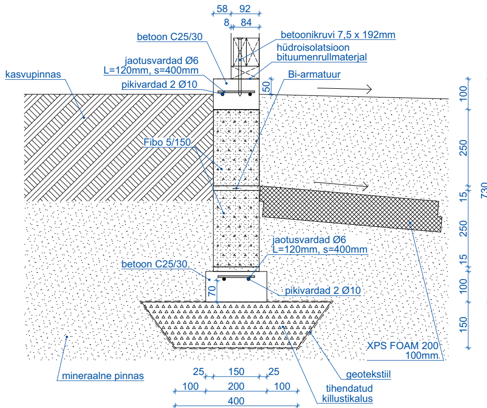
Vundamendi lõige M 1:10
