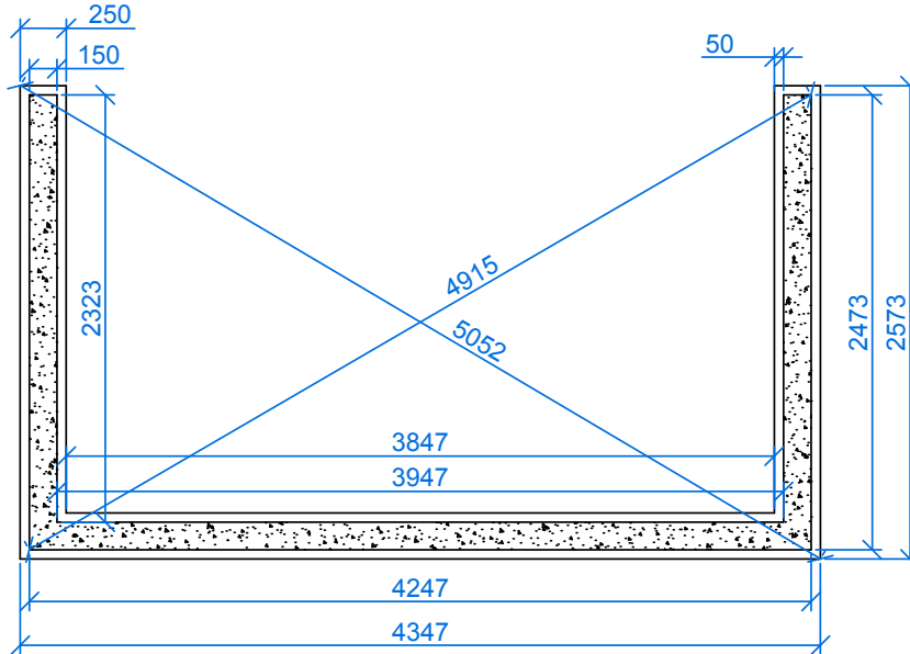
Vundamendi Plaan M 1:40
