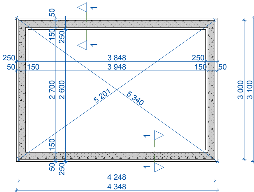
Vundamendi plaan M 1:50
